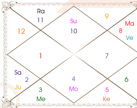
Shastiamsa Chart
