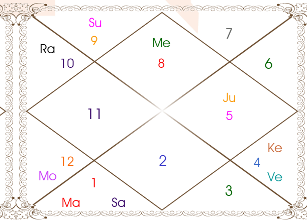
Shastiamsa Chart
