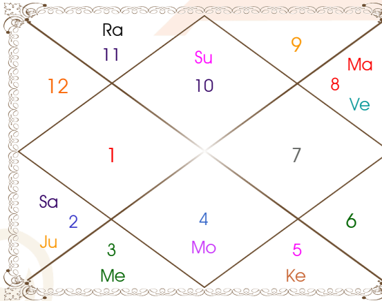
Shastiamsa Chart
