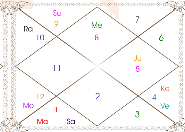
Shastiamsa Chart
